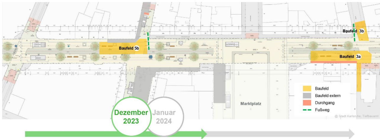
Abbildung 1: Baufelder Jahreswende 2023/2024
